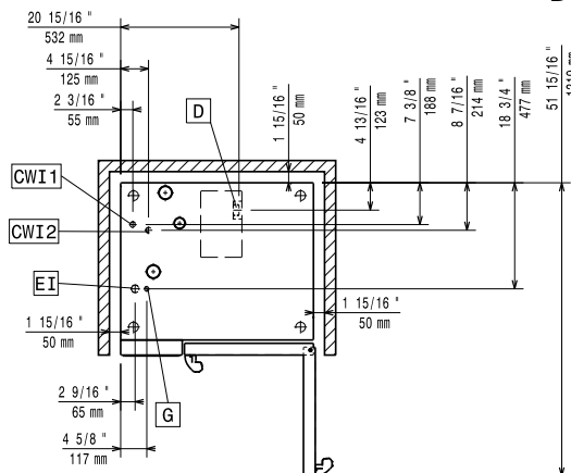
Dessus
